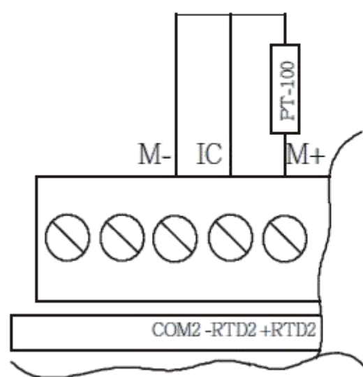
PT-100 Input
