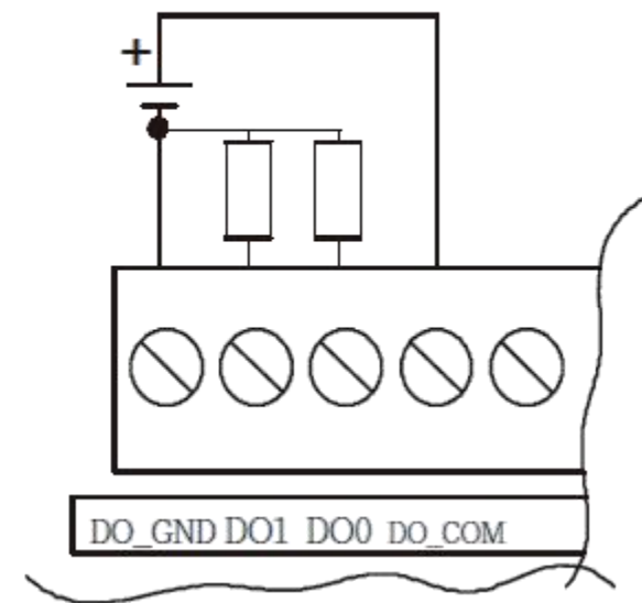
5190D/5190 Output
